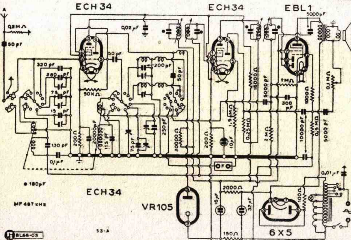
Lo schema elettrico del mod. R 851
